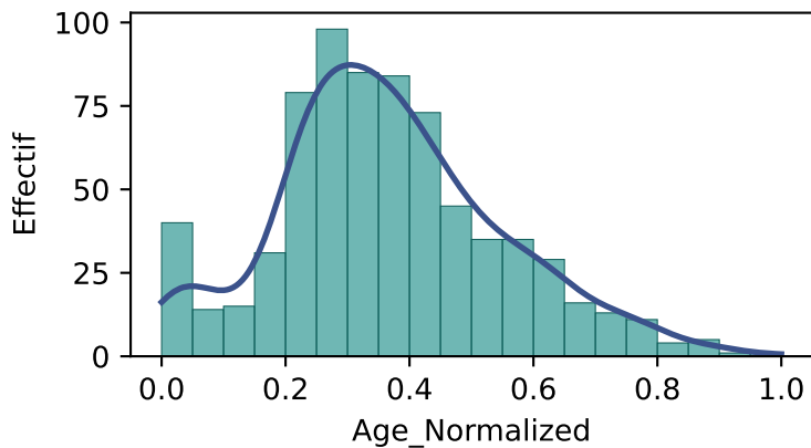
(c) Normalisation
